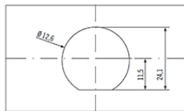
Frontplattenausschnitt
