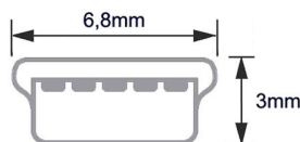
USB MINI B
